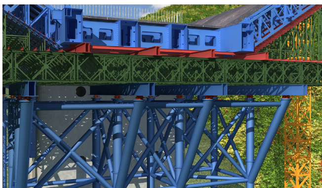
落地钢支架
